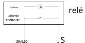
GS (señal de arranque del generador diésel)
